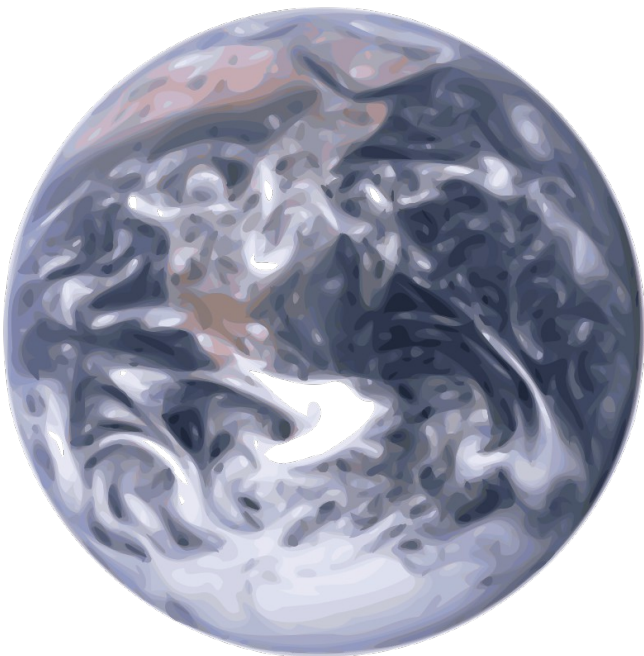
Earth
