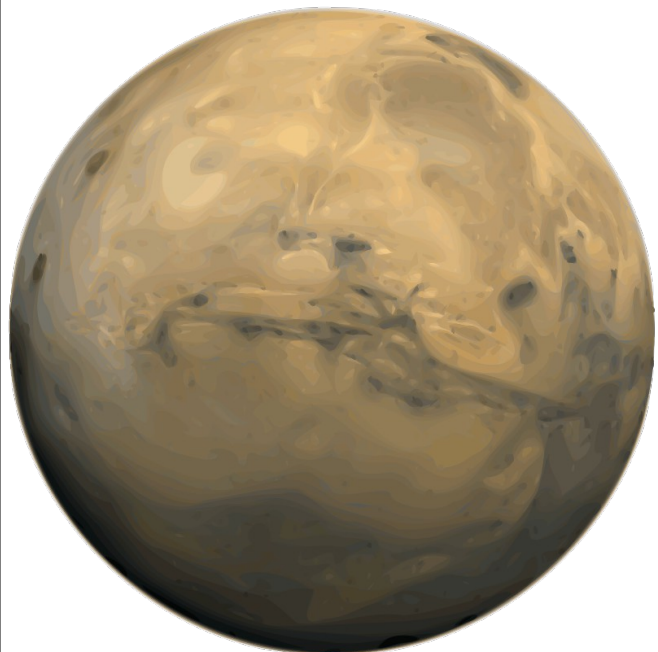
Mars
