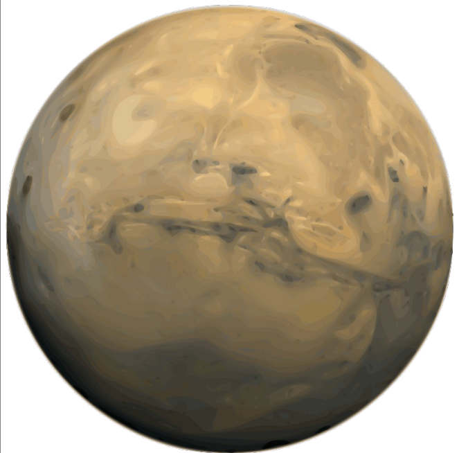
Mars
