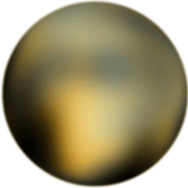
Pluto
