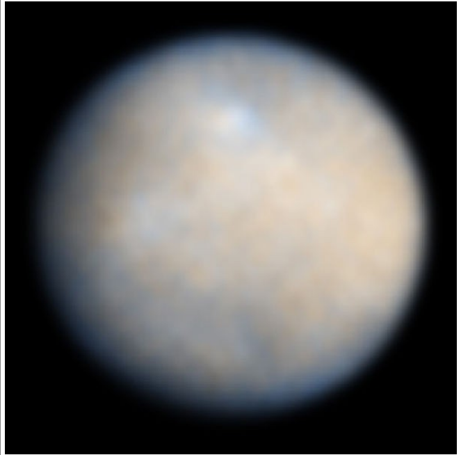
Ceres
