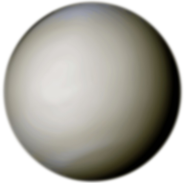
Venus
