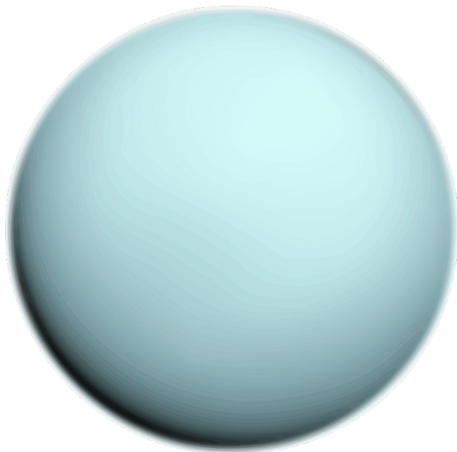
Uranus
